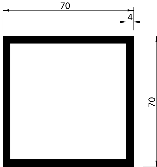
Stütze 70x70x4
