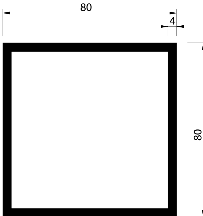
Stütze 80x80x4
